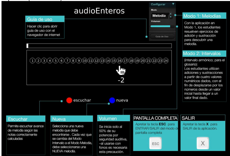
Figura 2. Pantalla principal del módulo AudioEnteros (AE).
